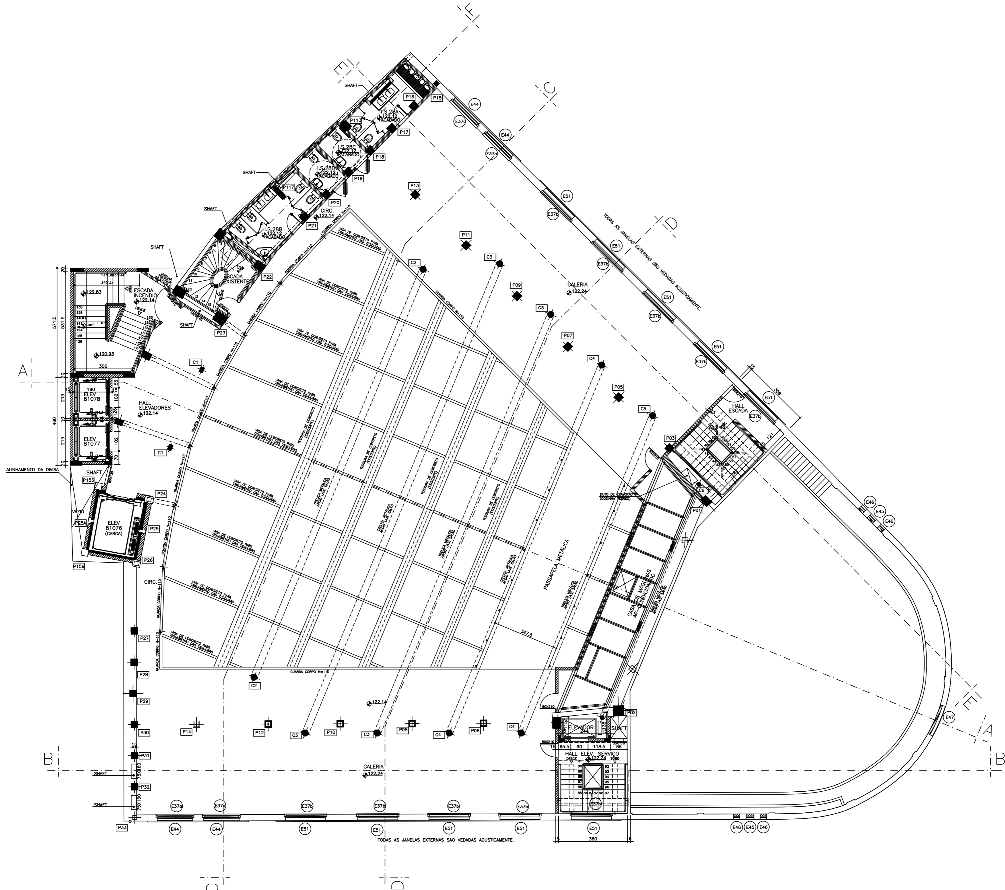
PLANTA 6º ANDAR – GALERIAS escala 1/75
